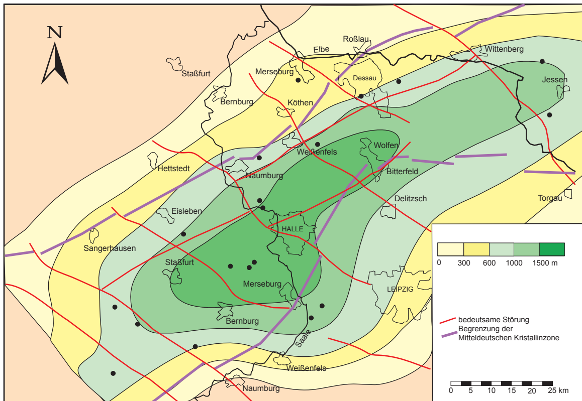
Abb. 30.12 Potentielle Verbreitung und Mächtigkeit von Schichtenfolgen des Permokarbons im Bereich der nordöstlichen Saale-Senke (nach I. RAPPILBER 2003)
