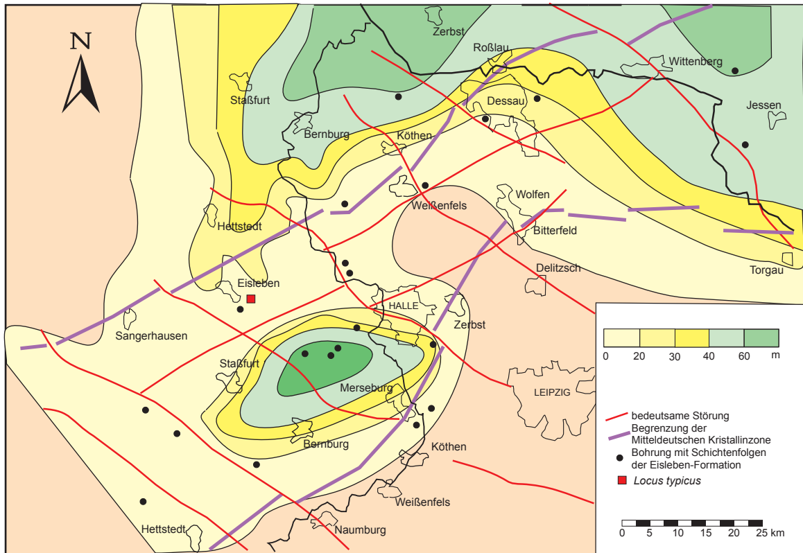
Abb. 30.11 Potentielle Verbreitung und Mächtigkeit von Schichtenfolgen der Eisleben-Formation im Bereich der nordöstlichen Saale-Senke (nach I. RAPPSILBER 2003)
