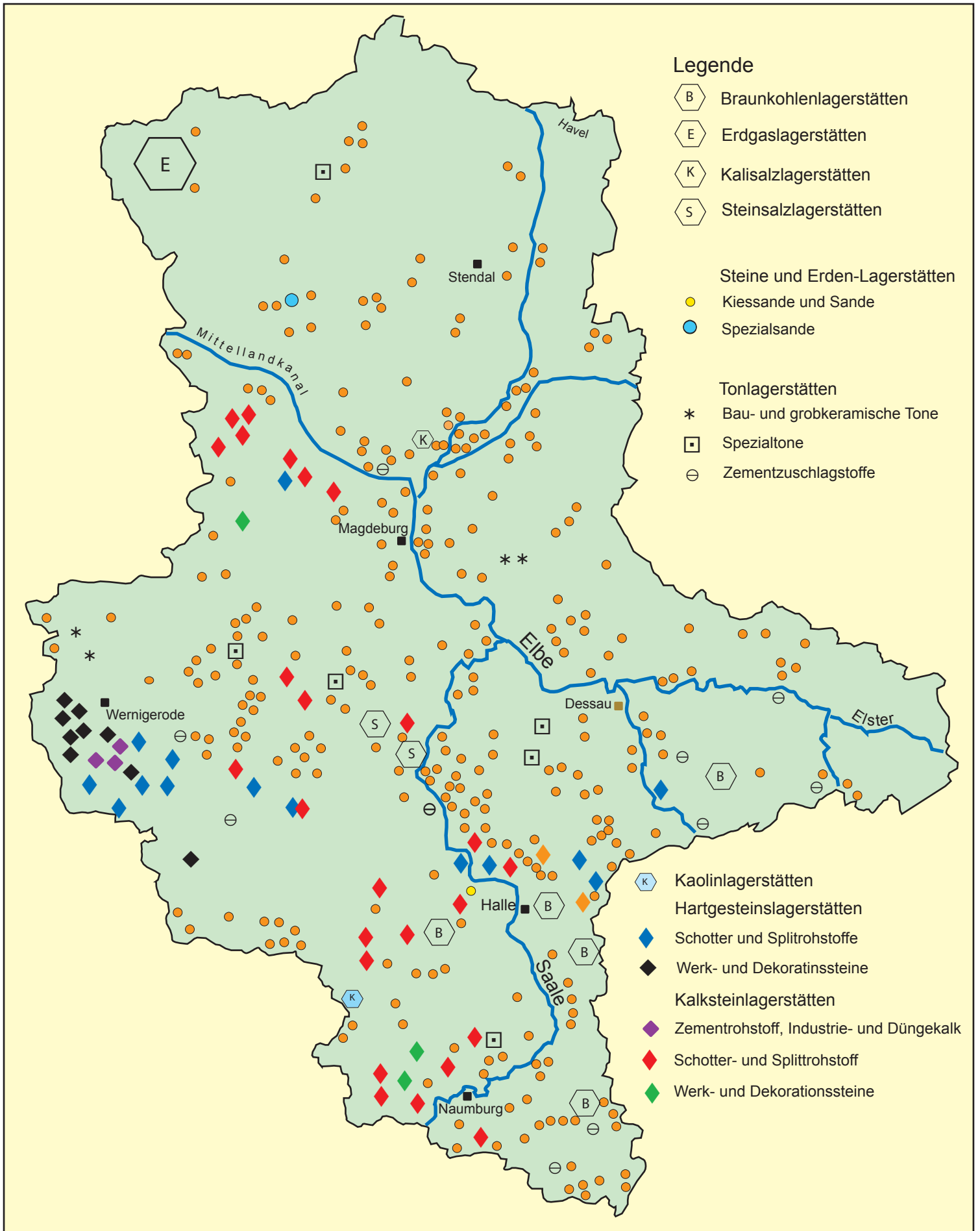
Abb. 30.13 Schematisierte Lagerstättenkarte von Sachsen-Anhalt
