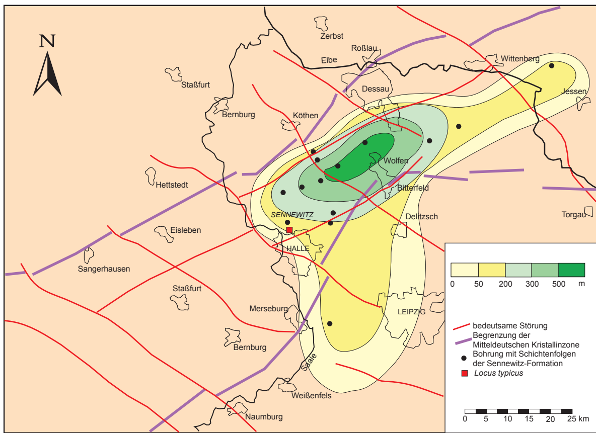
Abb. 30.8 Potentielle Verbreitung und Mächtigkeit von Schichtenfolgen der Sennewitz-Formation im Bereich der nordöstlichen Saale-Senke (nach I. RAPPILBER 2003)
