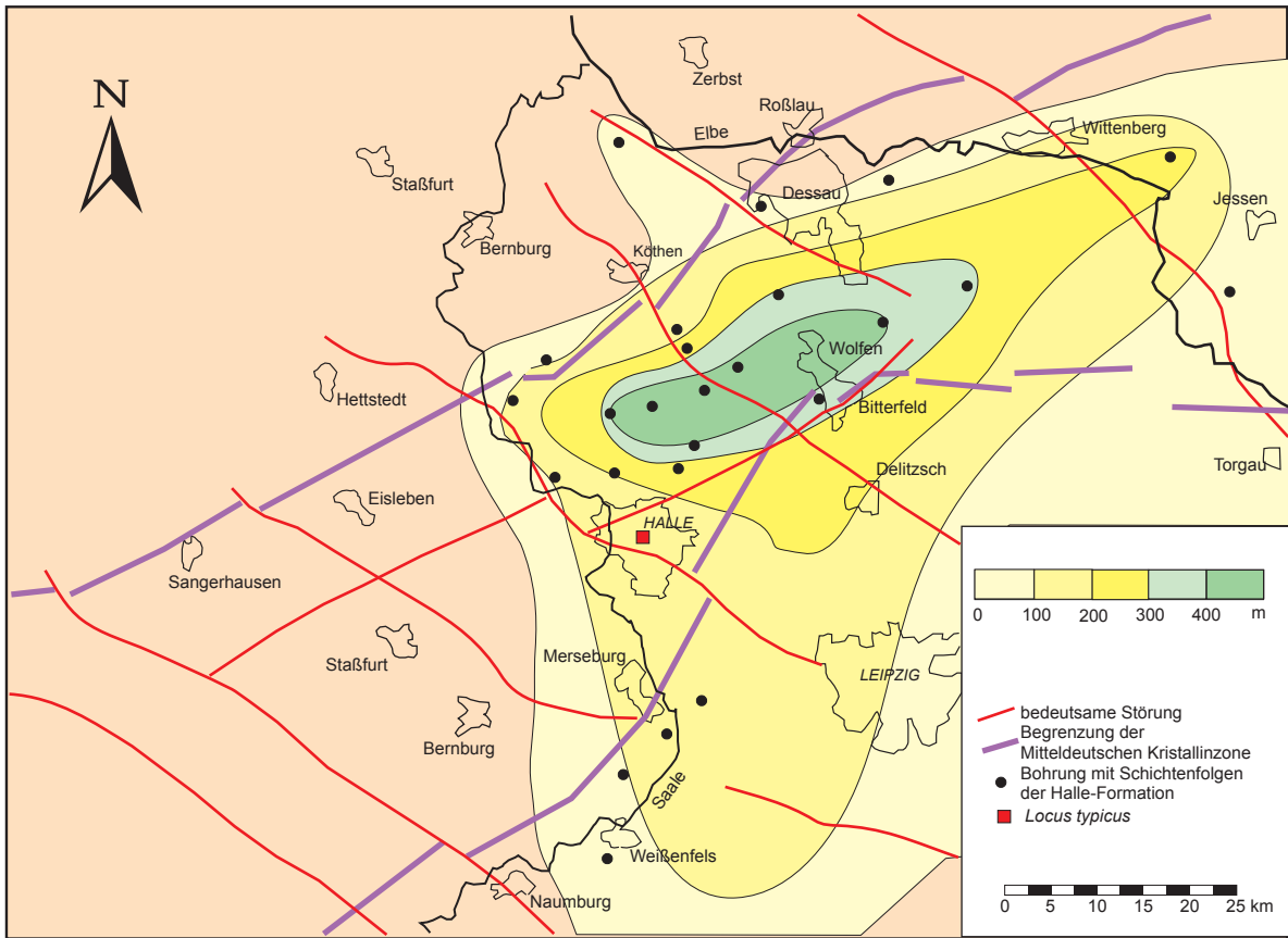
Abb. 30.7 Potentielle Verbreitung und Mächtigkeit von Schichtenfolgen der Halle-Formation im Bereich der nordöstlichen Saale-Senke (nach I. RAPPILBER 2003)
