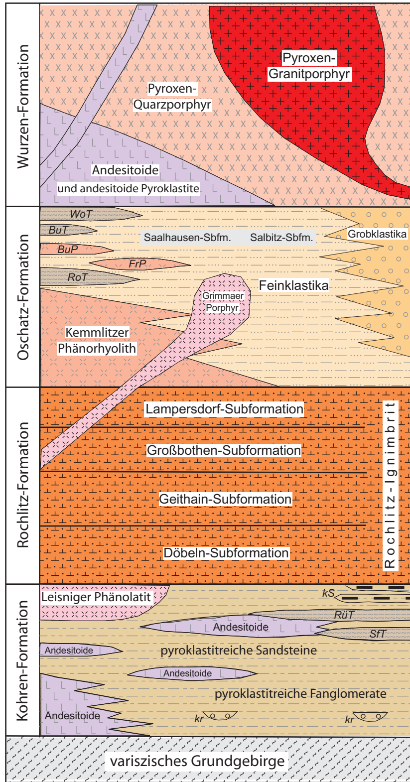
Abb. 31.2 Generalisiertes Normalprofil des Rotliegendes im Bereich des Nordwestsächsischen Eruptivkomplexes
