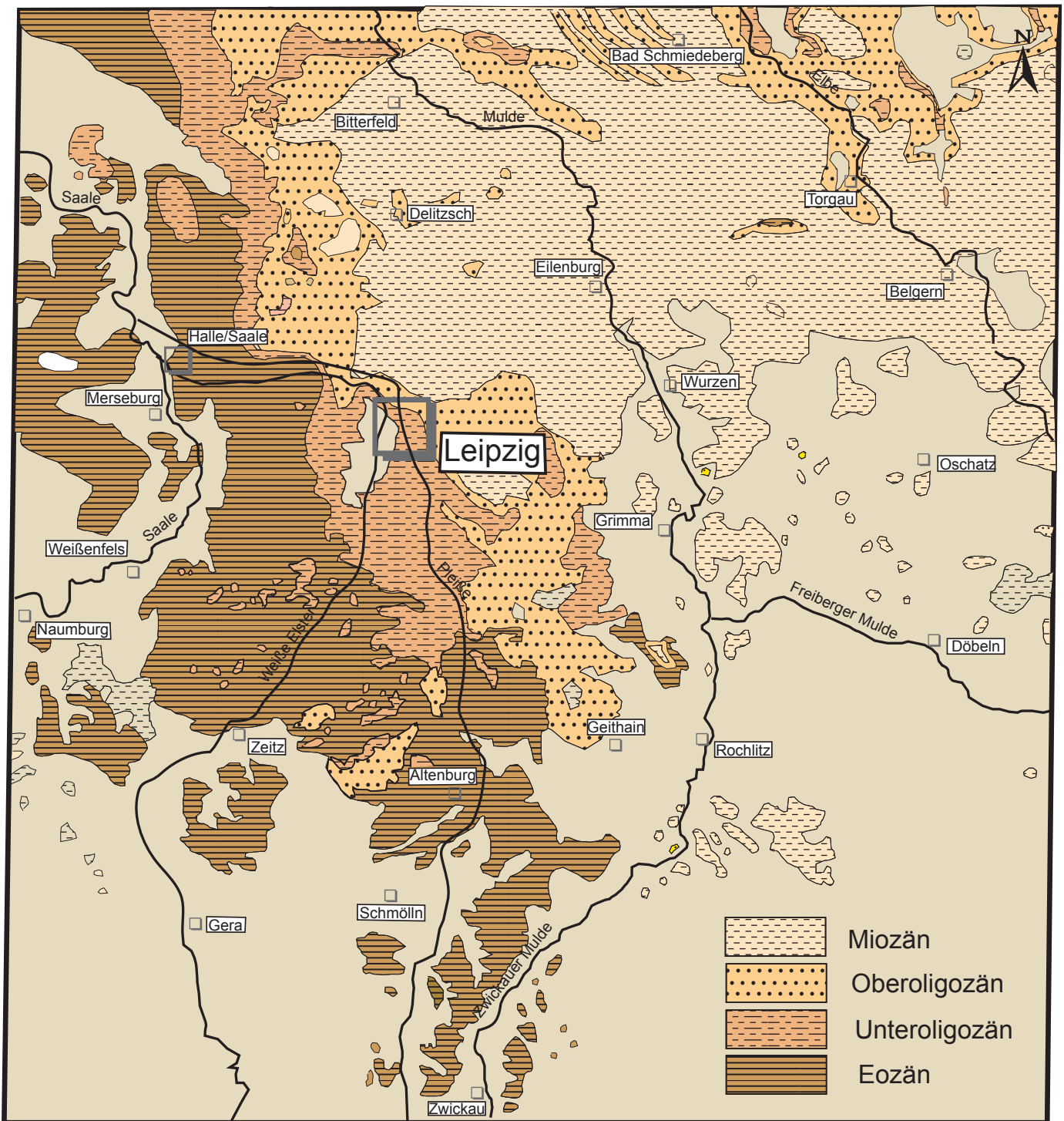
Abb. 31.5 Verbreitung von Schichtenfolgen des Tertiär im Bereich Nordwestsachsens und angrenzender Gebiete (nach L. EISSMANN 1995; A. BERKNER & P. WOLF 2004)
