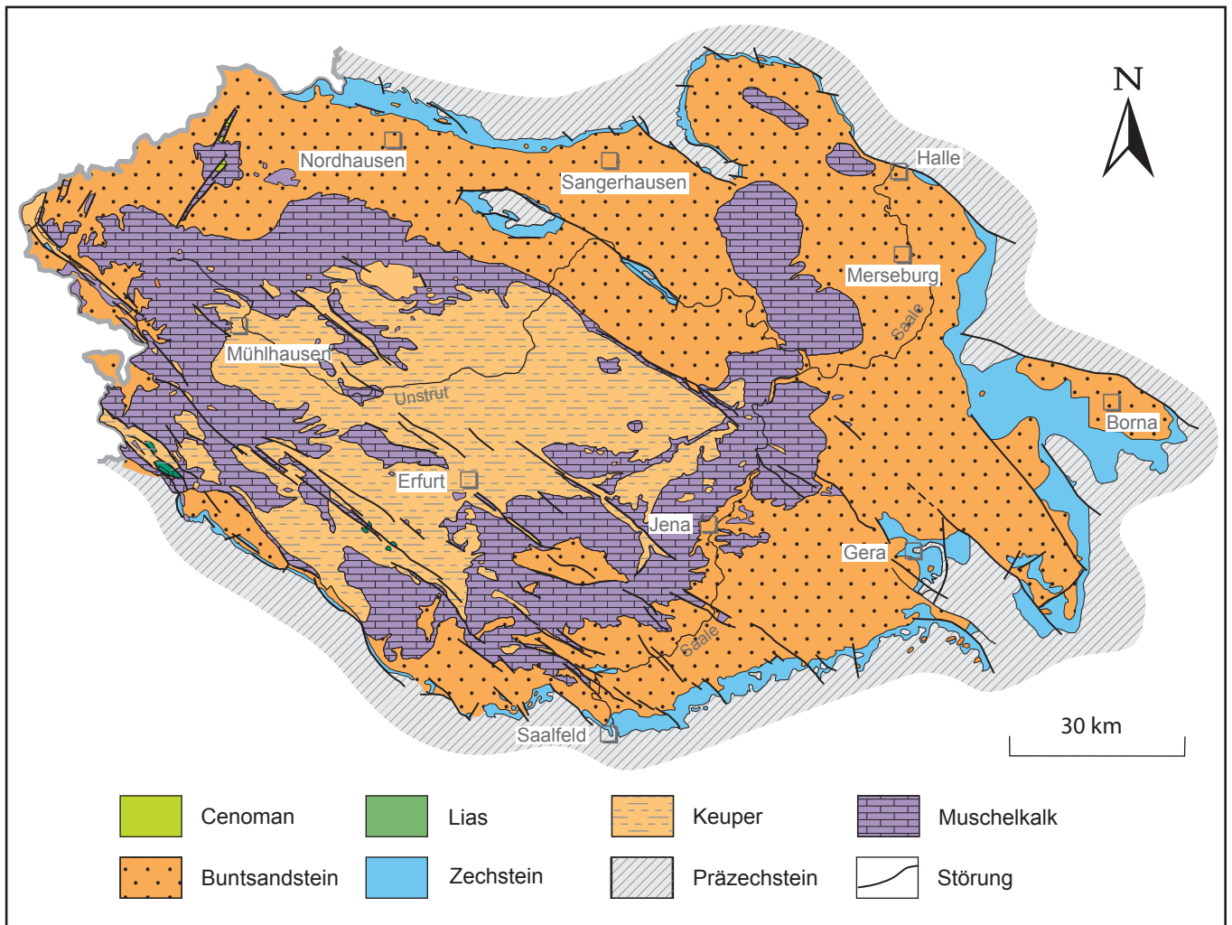
Abb. 32 Geologie des Thüringer Beckens sensu lato Darstellung ohne känozoische Bildungen (nach R. MUSSTOW 1990; P. PUFF 1994; G. SEIDEL et al. 2002)
