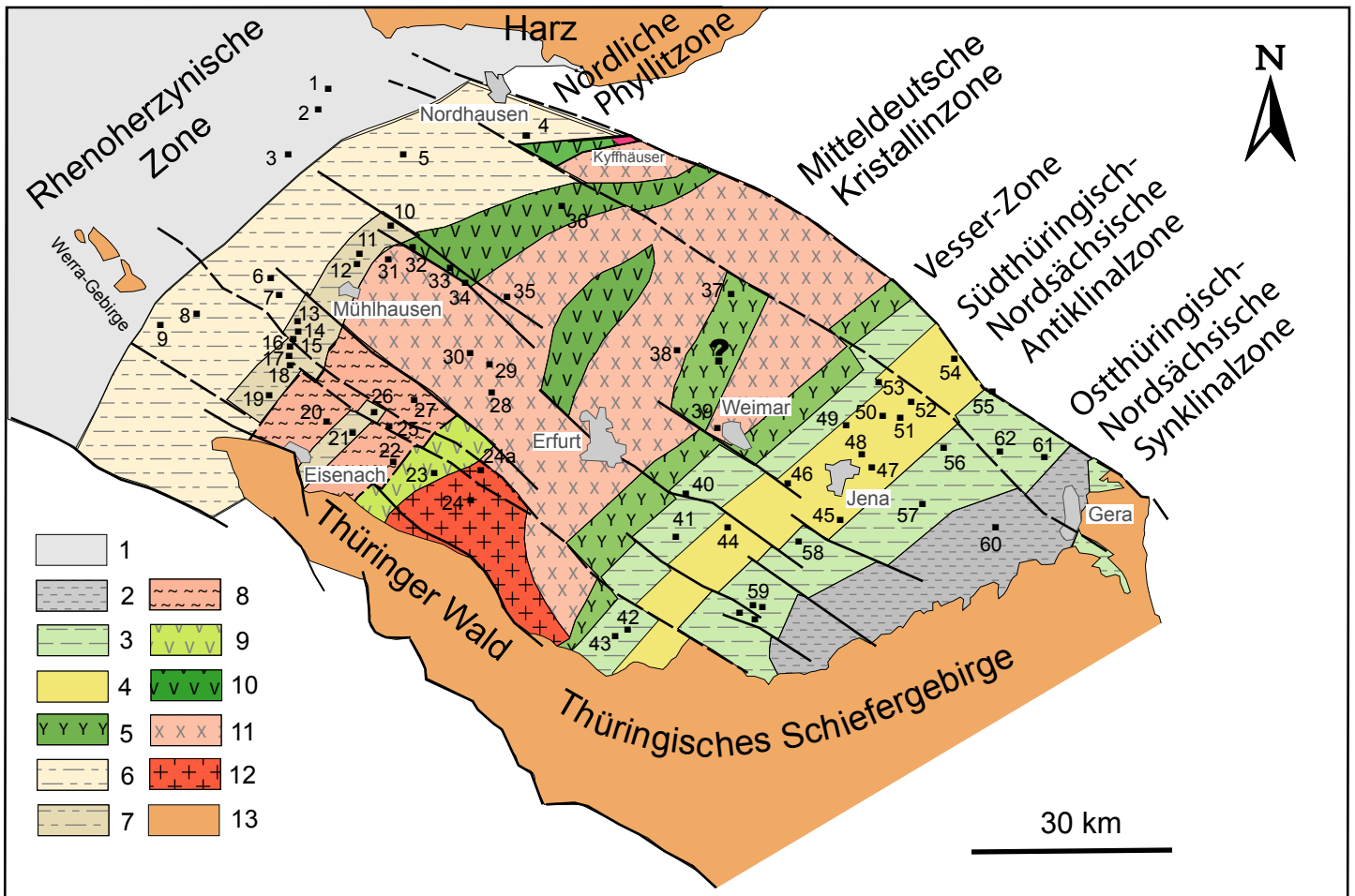
Abb. 32.4 Der prä-silesische Untergrund des Thüringer Beckens
