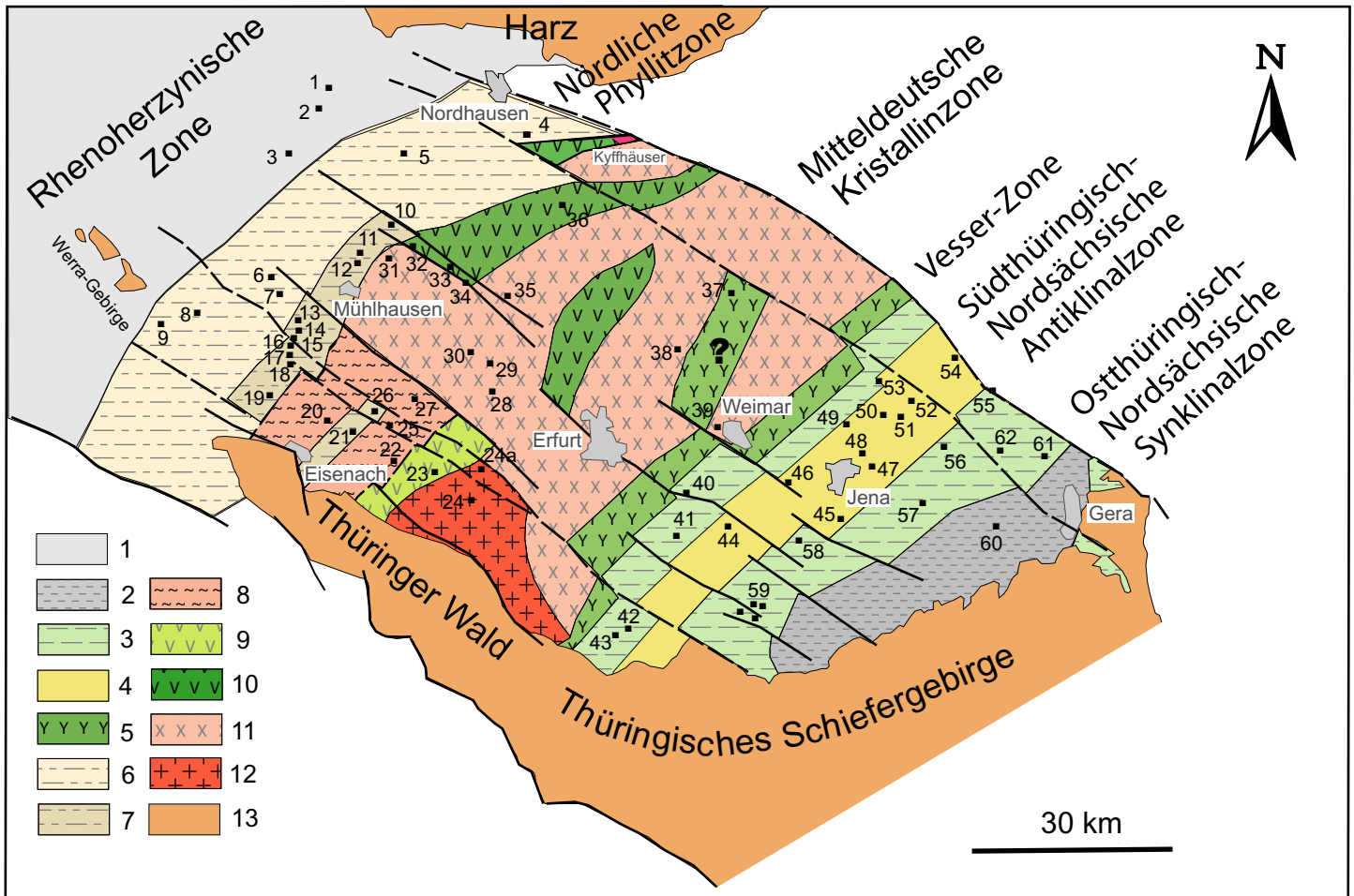
Abb. 32.4 Der präsilicische Untergrund des Thüringer Beckens
