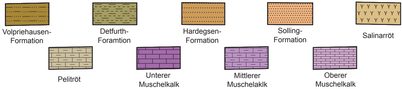
Abb. 32.6 Geologie des "Tannrodaer Gewölbes" im Südostteil des Thüringer Beckens (nach G. SEIDEL et al. 2002)
