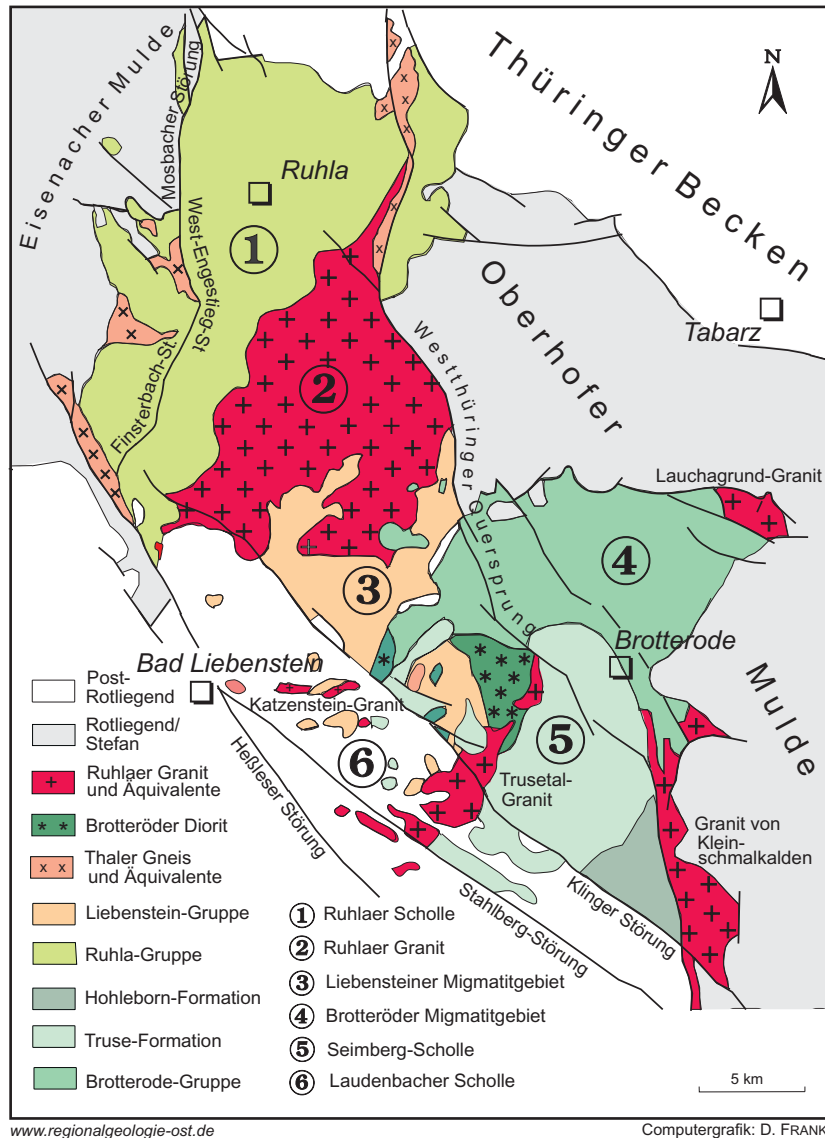
Abb. 33.2 Geologie des Ruhlaer Kristallins
