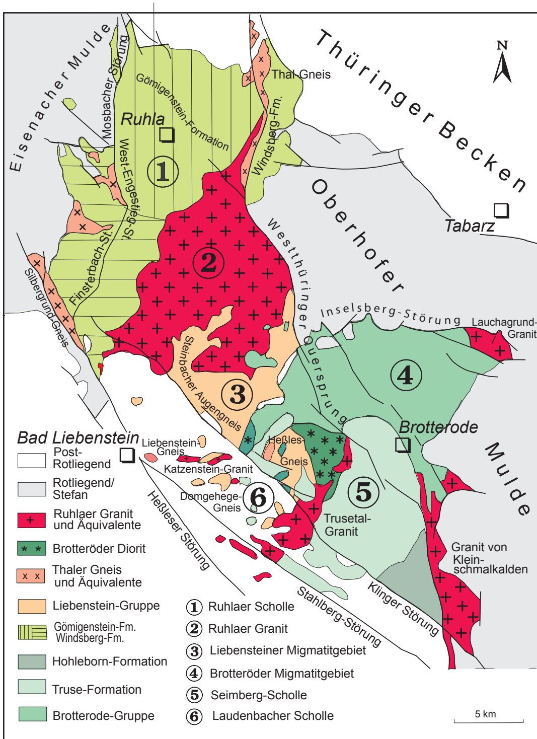
Abb. 33.2 Geologie des Ruhlaer Kristallins
