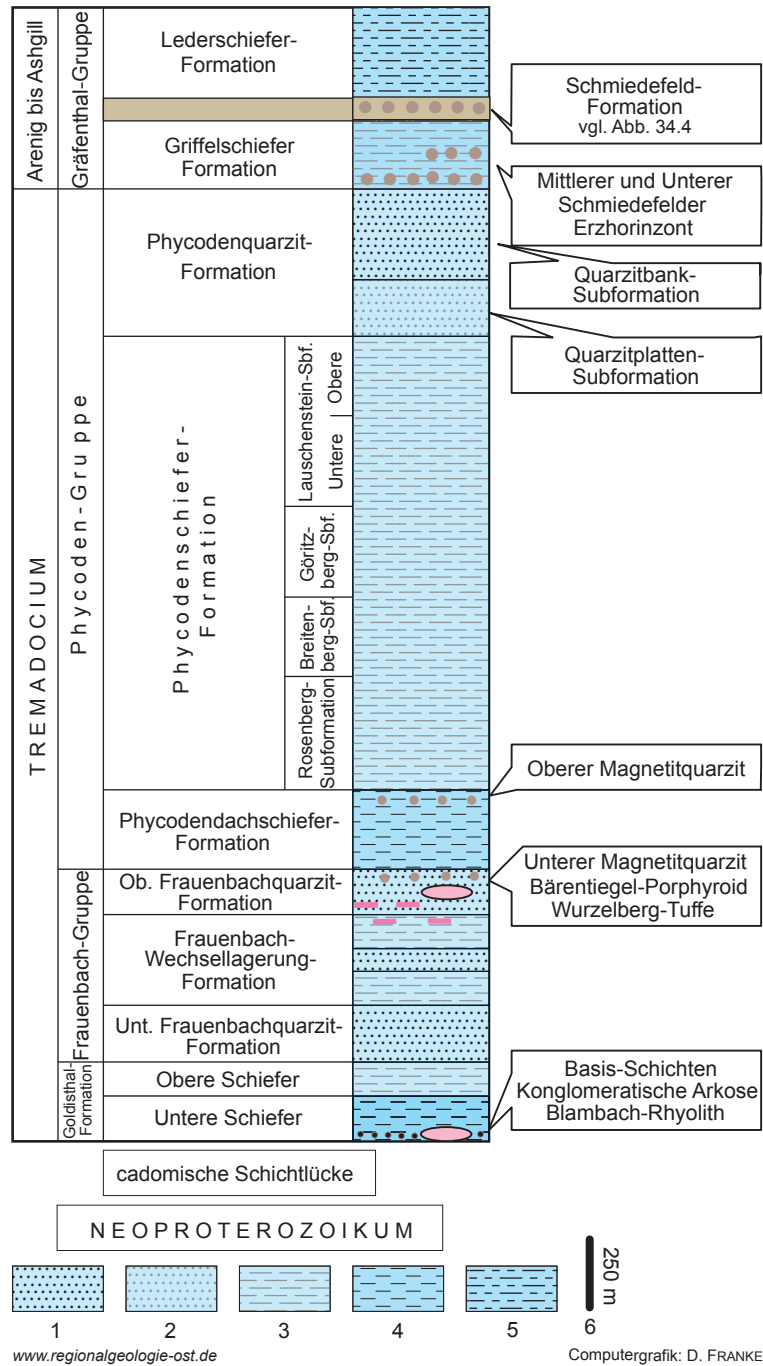
Abb. 34.3 Stratigraphie des Ordovizium an der Südostflanke des Schwarzbunger Antiklinoriums
