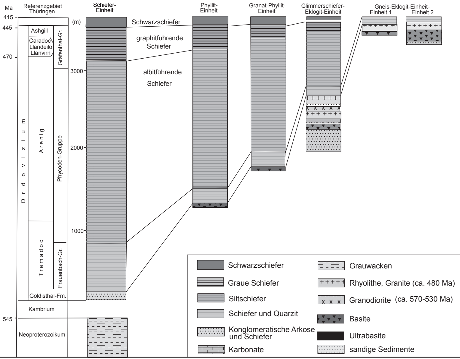
Abb.. 36.17 Entwurf einer tektonostratigraphischen Korrelation von ordovizischen Ablagerungen des Schwarzburger Antiklinoriums mit metamorphen Einheiten des Erzgebirgs-Antiklinoriums
