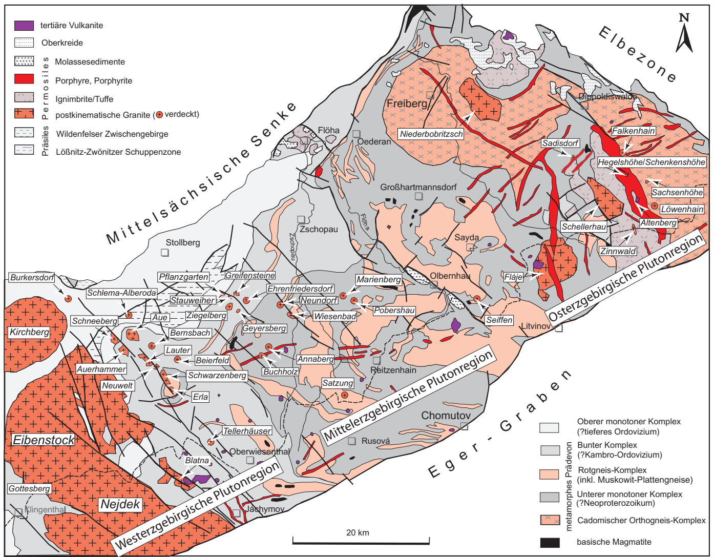
Abb. 36.2 Variszische Granite des Erzgebirgs-Antiklinoriums
