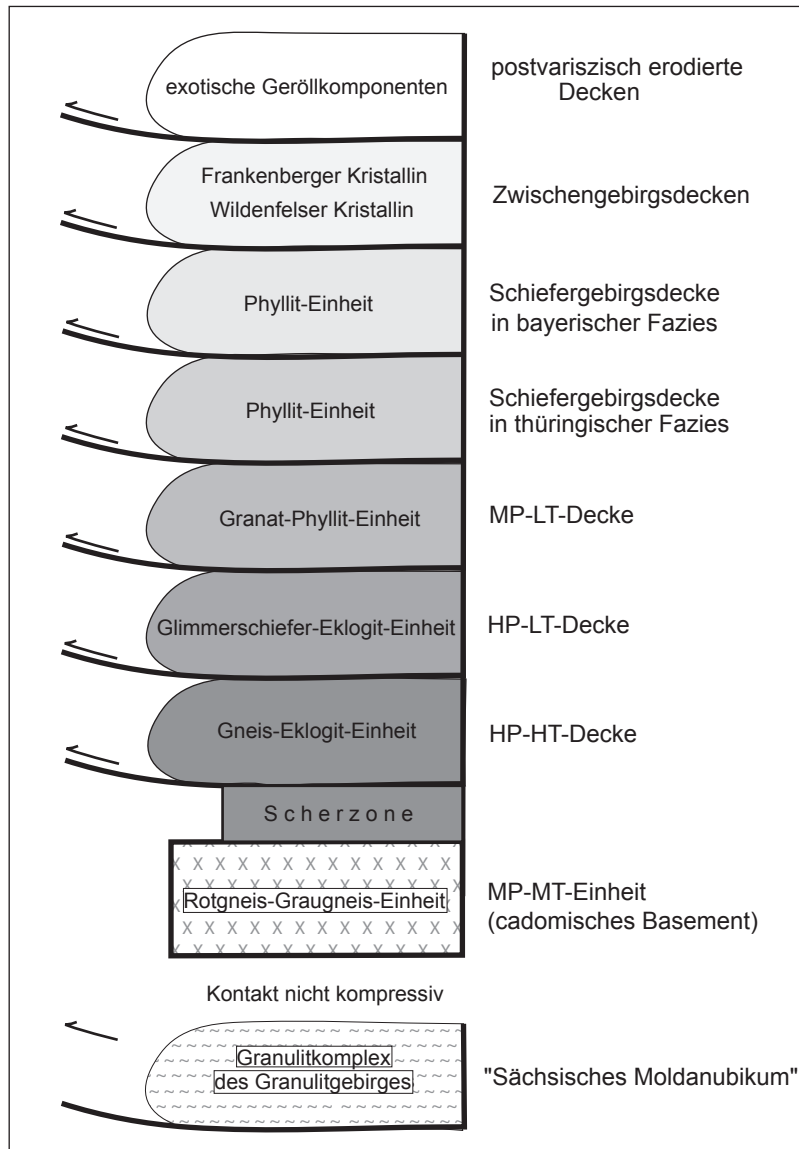
Abb. 36.10 Modell der Deckenstapelung im östlichen Saxothuringikum (nach K. RÖTZLER 1995; U. KRONER & U. SEBASTIAN 1997; B. MINGRAM & K. RÖTZLER 1999; K. RÖTZLER & B. PLESSSEN 2010)
