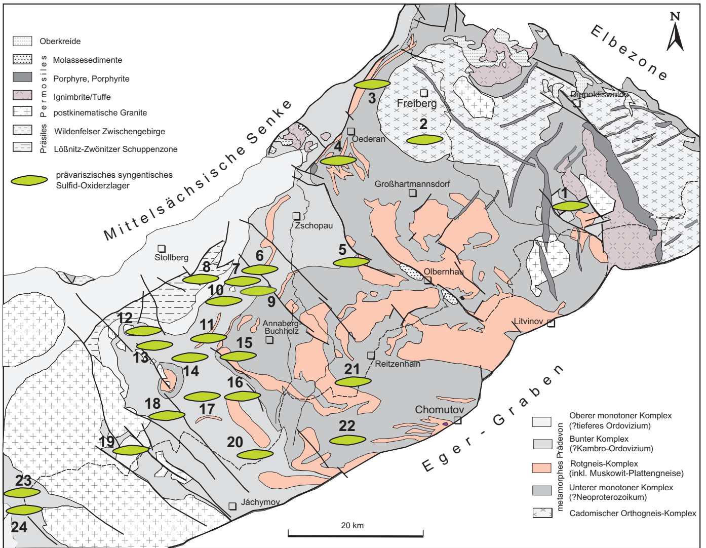
Abb. 36.7 Regionale Verbreitung prävariszischer syngenesischer Sulfid-Oxidierzlager im Erzgebirge (Auswahl)
