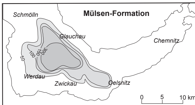
Abb. 37.1.1 Isopachen des Rotliegend im Bereich der Vorerzgebirgs-Senke (nach H. BRAUSE & H.-J. BERGER 2006)
