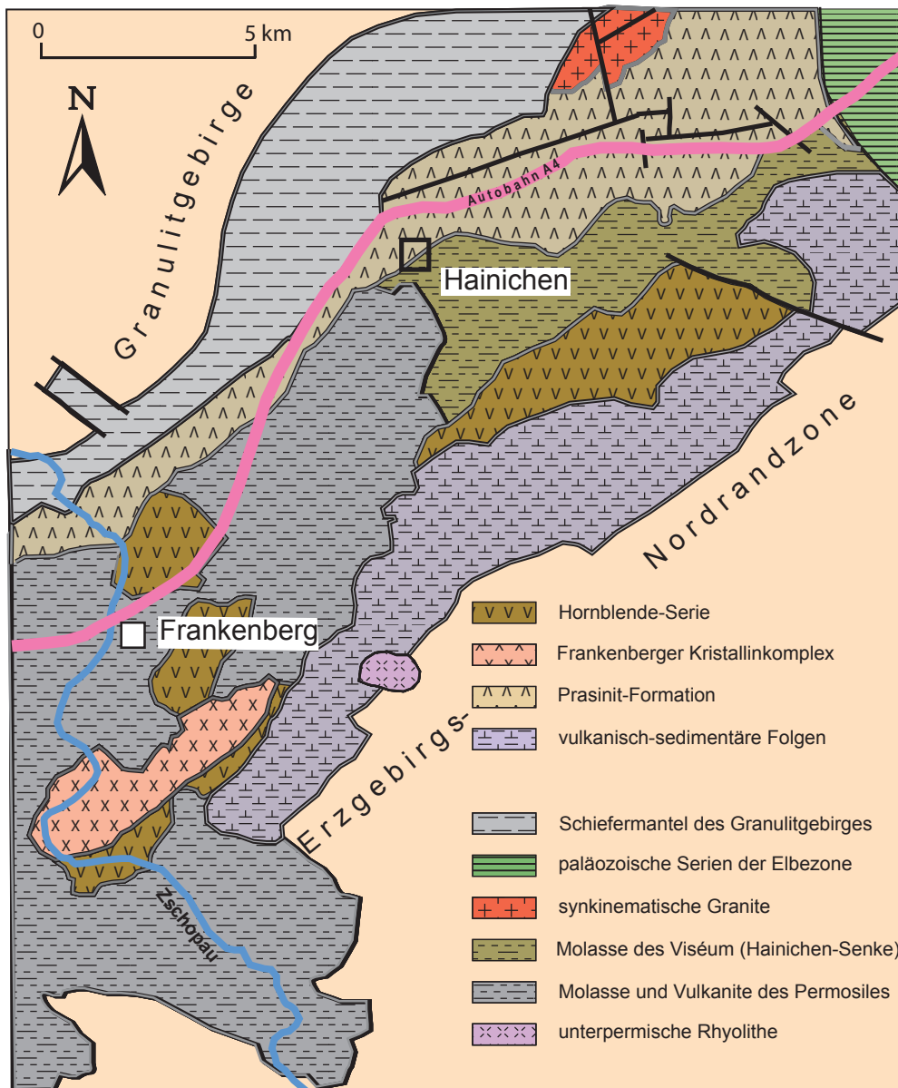
Abb. 38.1 Geologie des Frankenberger Zwischengebirges und angrenzender Einheiten
