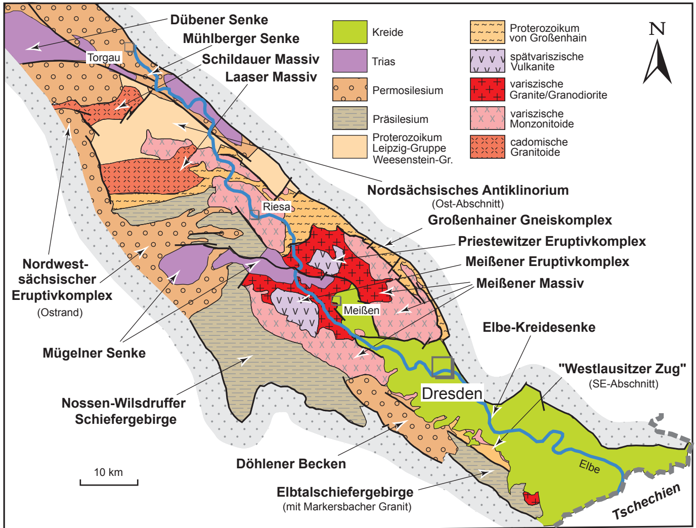
Abb. 39 Regionaleinheiten der sächsischen Elbezone Darstellung ohne känozoische Bildungen
