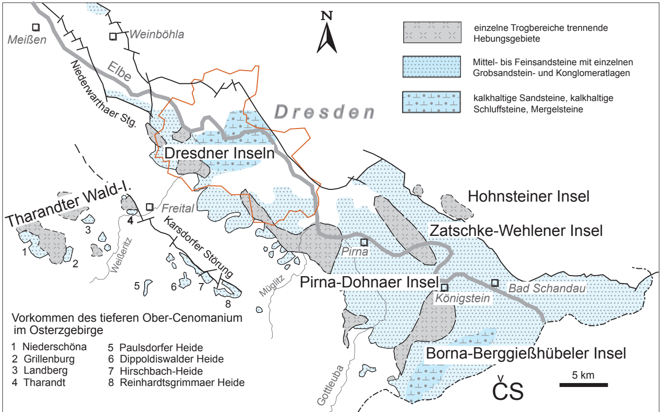
Abb. 39.2 Paläogeographie des Ober-Cenomanium der Elbtalkreide (hier: Oberhäslich-Formation, Mobschatz-Formation) mit differenzierter Beckenkonfiguration bei annähernd homogener Lithofaziesentwicklung
