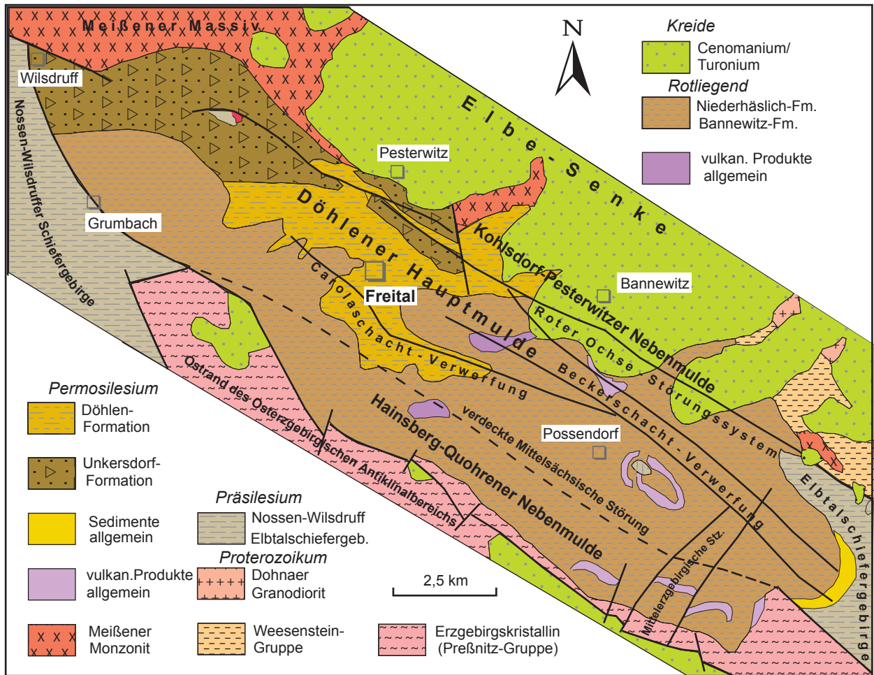
Abb. 39.5 Geologie des Döhlener Beckens Darstellung ohne känozoische Bildungen
