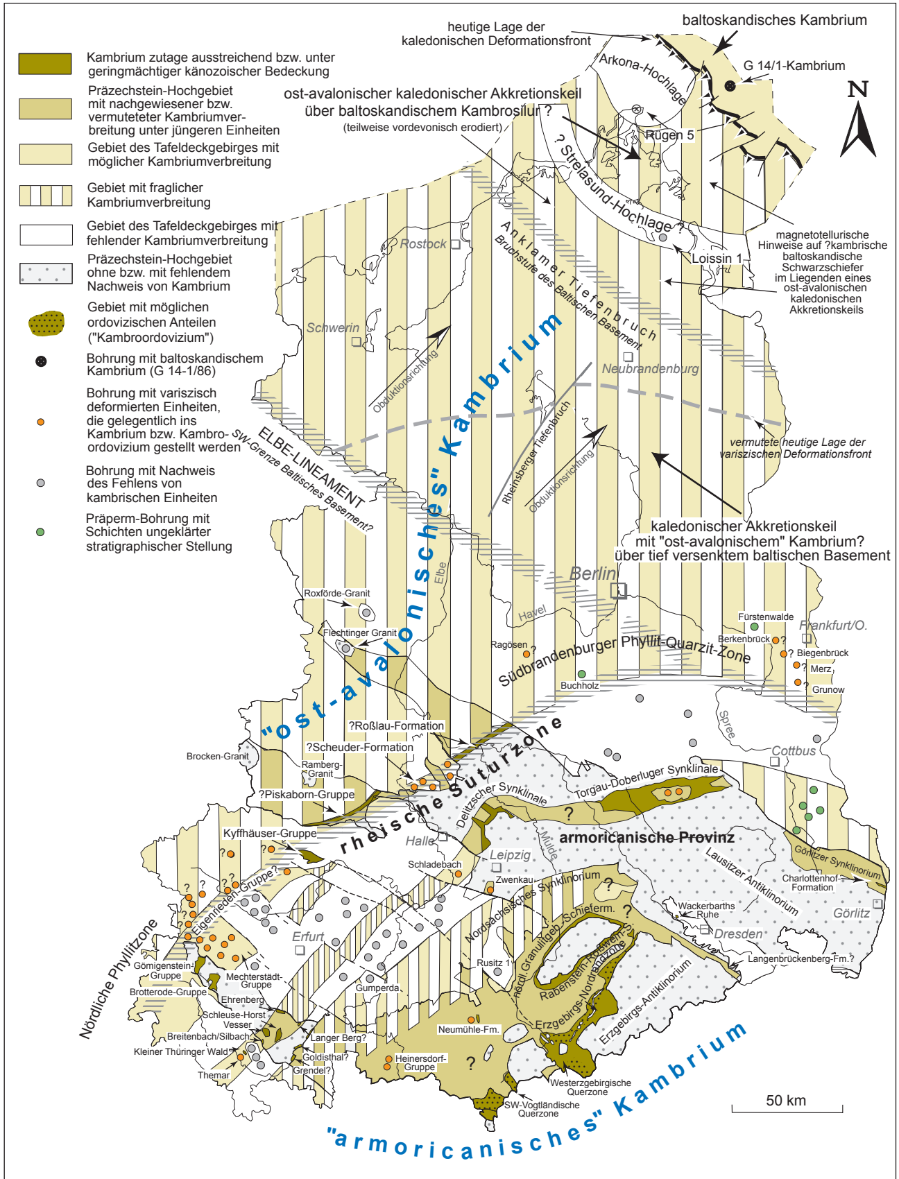
Abb. 4.1 Heutige Verbreitung von Ablagerungen des Kambrium (einschließlich ?Kambro-Ordovizium) in Ostdeutschland Die nach den derzeit gängigen plattentektonischen Modellen eingetragenen Suturezonen sind im Detail noch gering begründet
