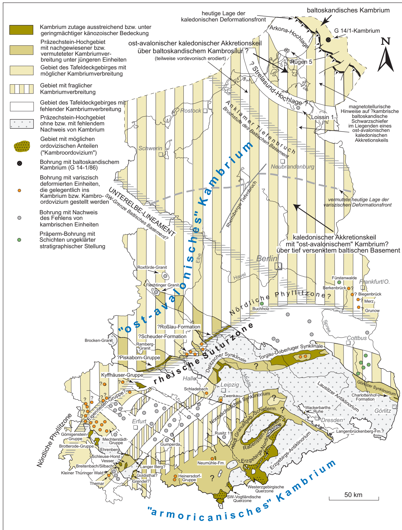
Abb. 4.1 Heutige Verbreitung von Ablagerungen des Kambrium (einschließlich ?Kambro-Ordovizium) in Ostdeutschland Die nach den derzeit gängigen plattentektonischen Modellen eingetragenen Suturezonen sind im Detail noch gering begründet
