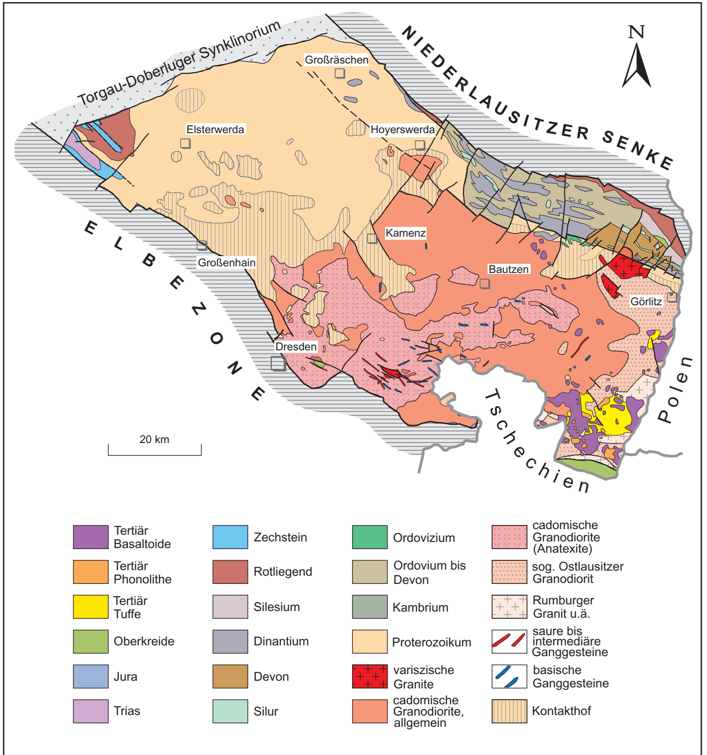
Abb. 40 Geologie des Lausitzer Antiklinoriums Darstellung ohne Sedimente des Känozoikum
