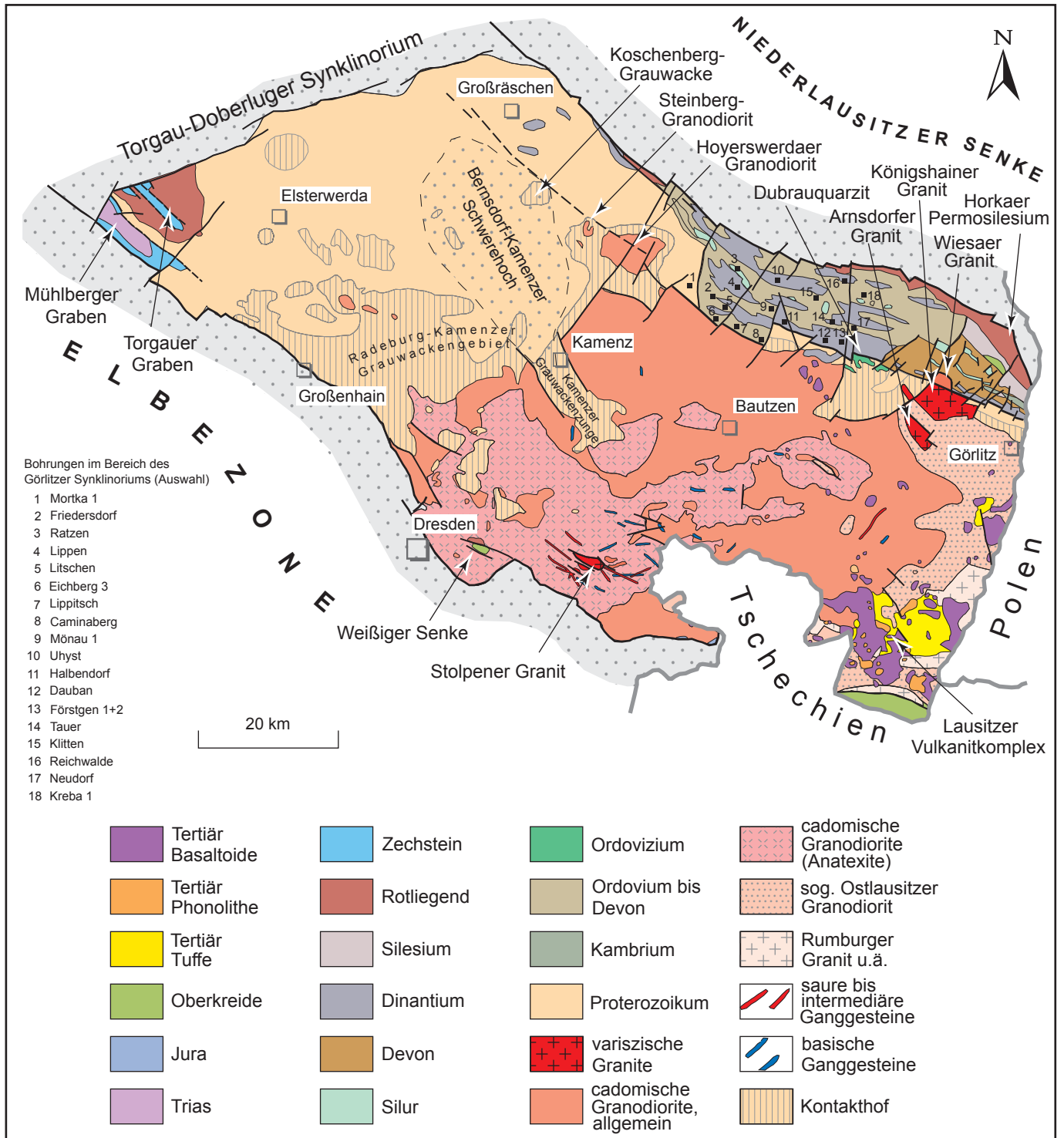
Abb. 40.2 Regionale Teilelemente im Bereich des Lausitzer Antiklinoriums Darstellung ohne Sedimente des Känozoikum
