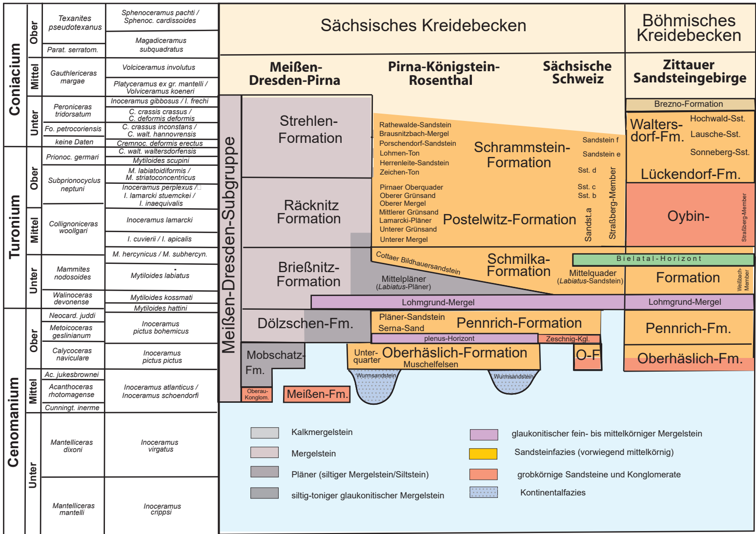
Abb. 40.5 Stratigraphie der Elbtal-Gruppe des Sächsisch-Böhmischen Kreidebeckens
