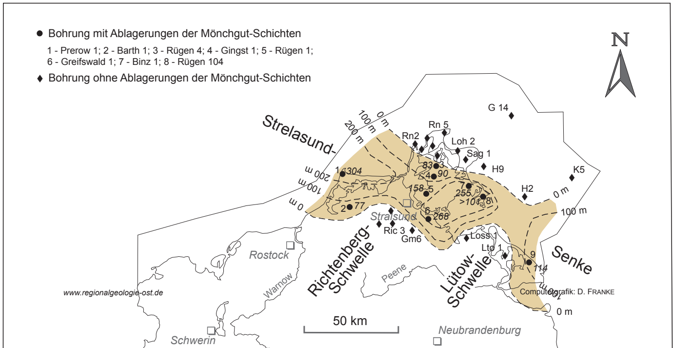
Abb. 9.2 Heutige Verbreitung von Ablagerungen des Karbon/Perm-Grenzbereichs (Mönchgut-Schichten) auf Rügen und dem angrenzenden Festland
