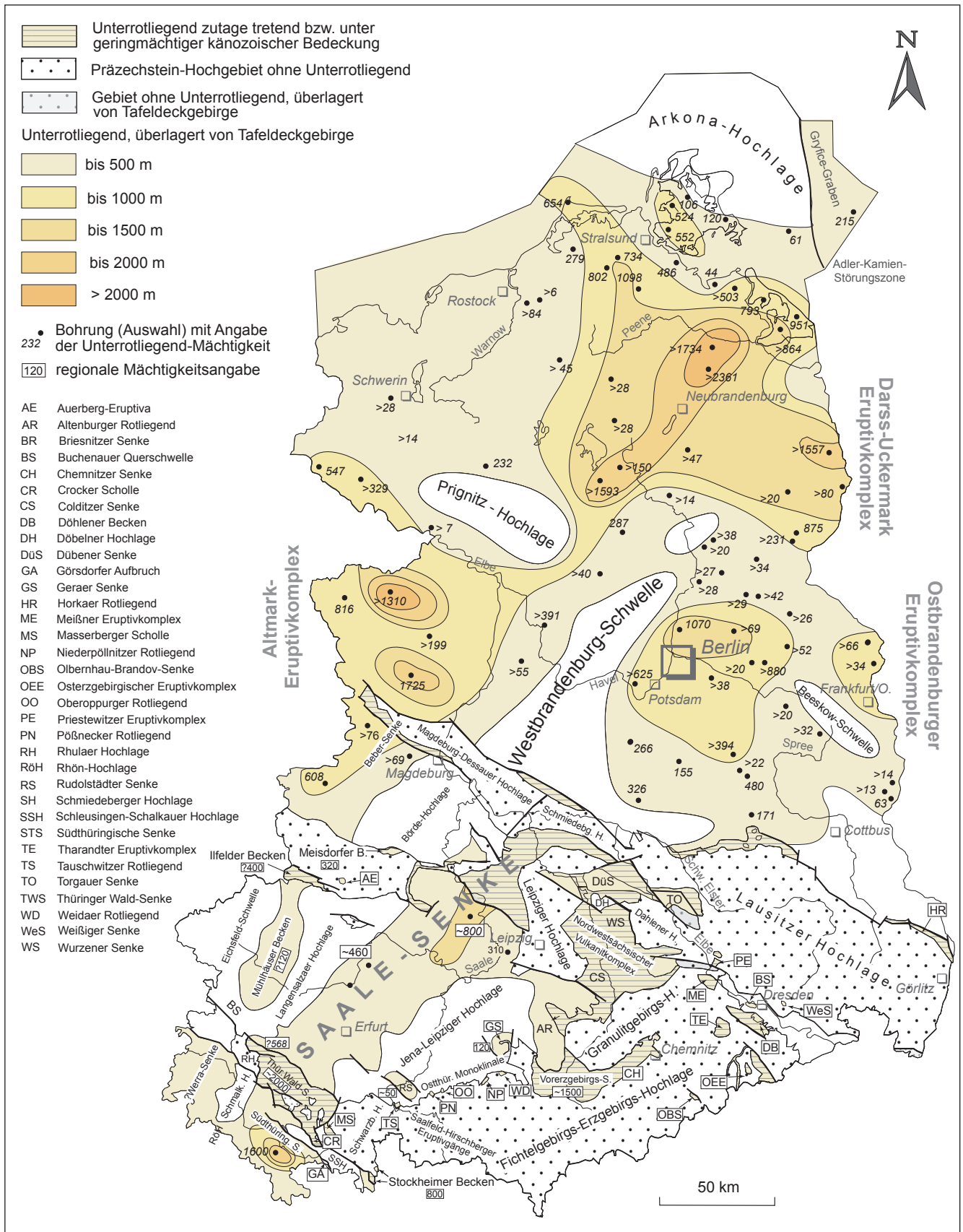
Abb. 9.3 Heutige Verbreitung von sedimentären und/oder vulkanogenen Einheiten des Unterrotliegend (einschließlich höchstem ?Stefanium) in Ostdeutschland
